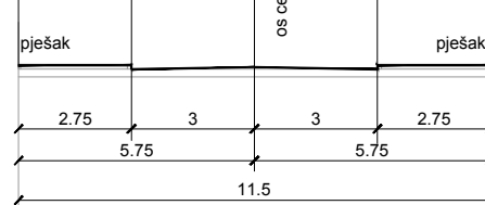
KARAKTERISTIČAN POPREČNI PRESJEK B
