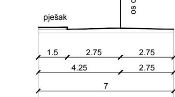
KARAKTERISTIČAN POPREČNI PRESJEK B
